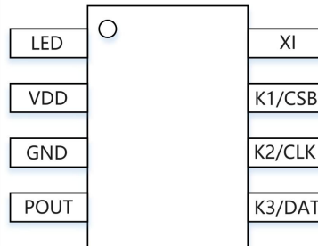
图 1 VI2150L/VI2157L 管脚示意图
