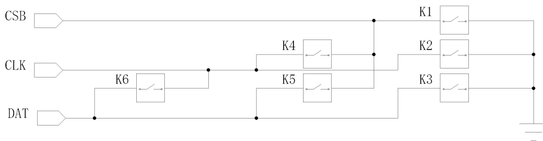
图 4 VI2150L/VI2157L 按键扫描示意图
