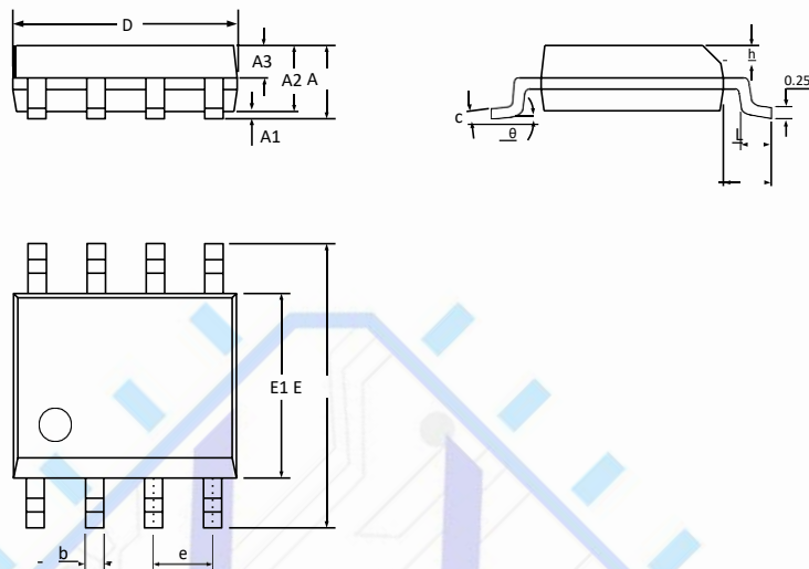
图 6 VI2150L/VI2157L 封装示意图
