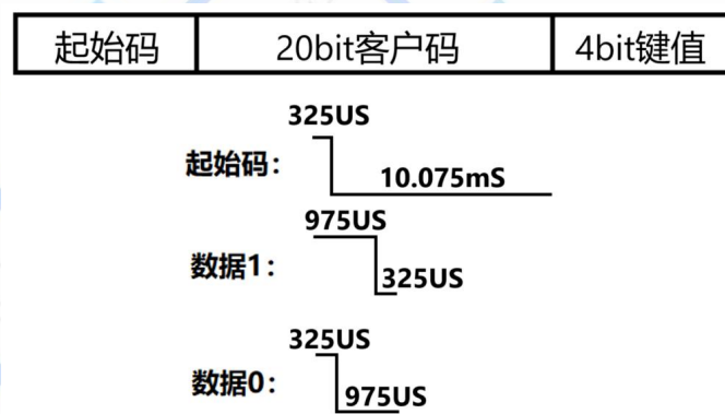
图 5 VI2150L/VI2157L 默认程序数据包定义及数据说明
