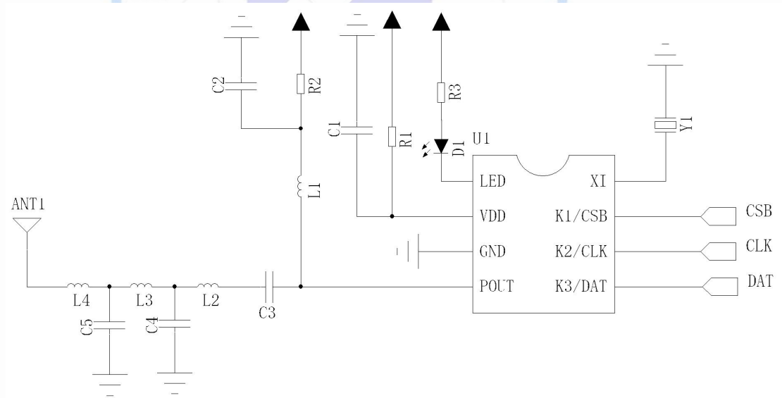
图 3 VI2150L/VI2157L 典型应用电路
