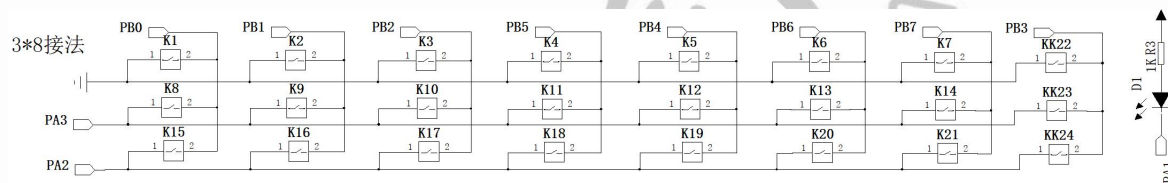
图 4 VM8852T 24 键应用电路按键部分
