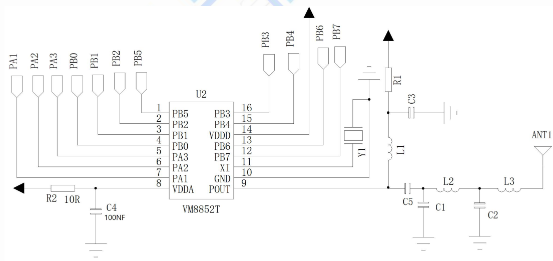
图 3 VM8852T 应用电路射频部分（天线匹配部分参数见表 6）
