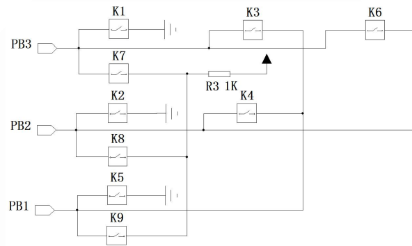
图 8 VM8806T 9 键应用电路按键部分
