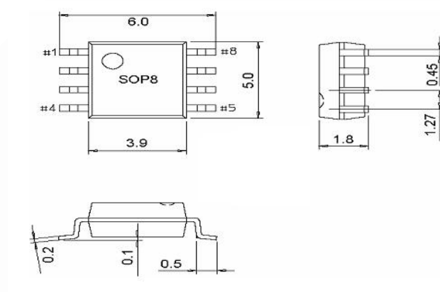
图 12 VM8806T SOP8 封装示意图
