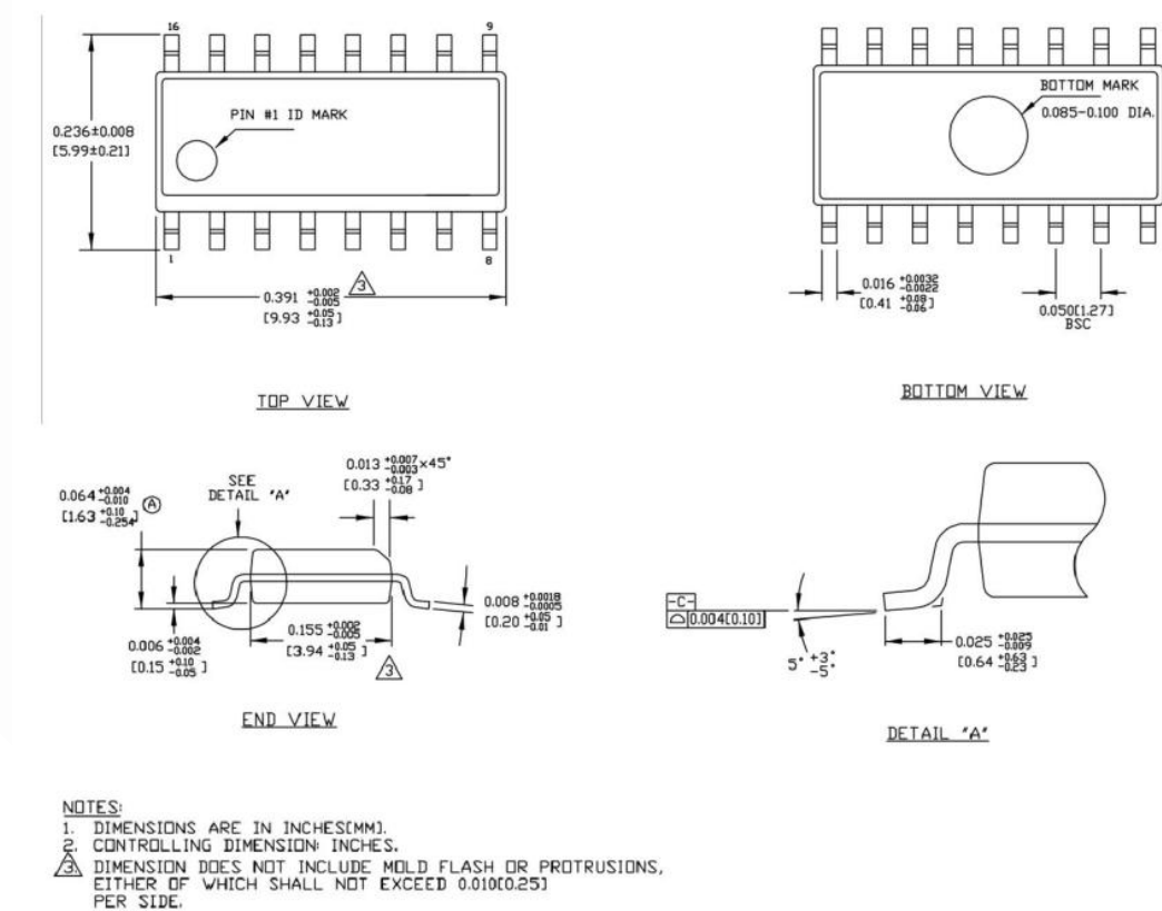
图 13 VM8852T SOP16 封装示意图
