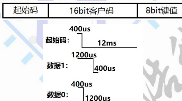
图 11 VM88XXT 默认程序数据包定义及数据说明
