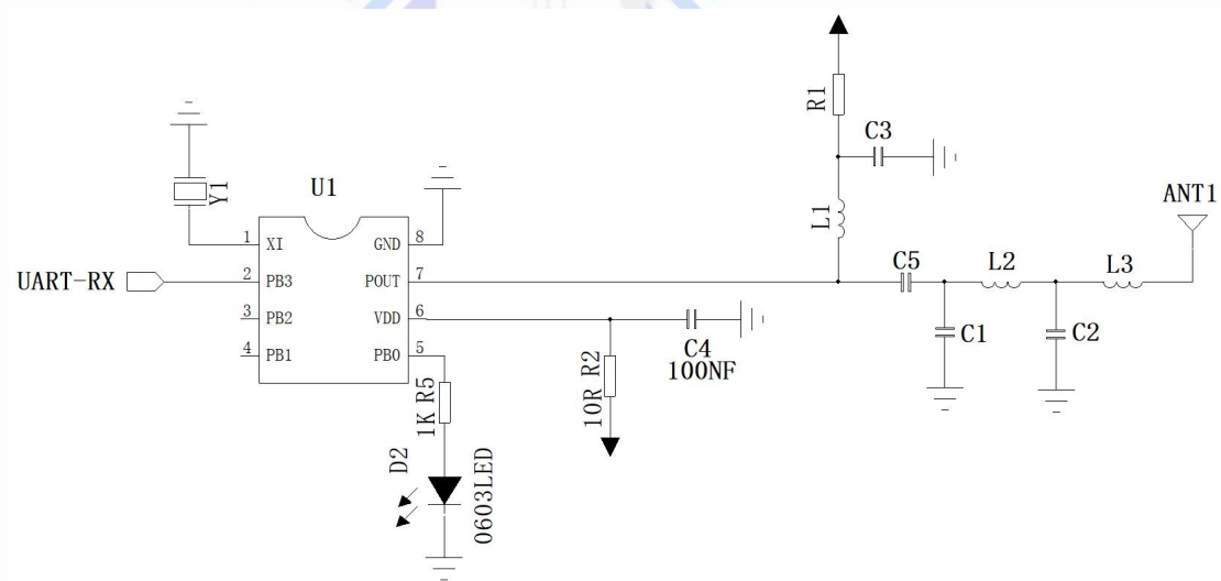
图 9 VM8806T 串口转 1527 应用电路图
