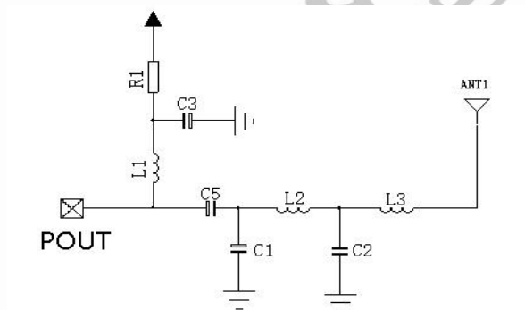
图 10 VM88XXT 天线匹配电路
