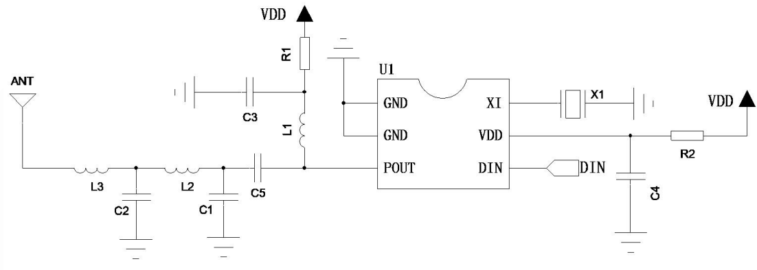
图 3 VI8855B 典型应用电路
