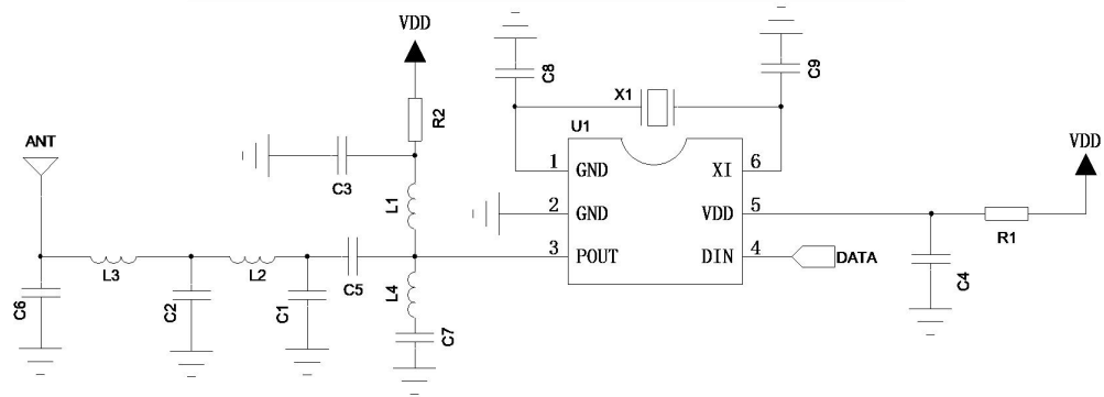
图 4 VI8855B 认证应用电路
