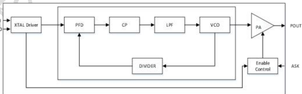
图 2 VI8805H 内部电路框架图
