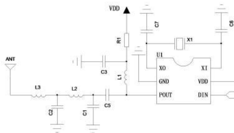
图 3 VI8805H 典型应用电路
