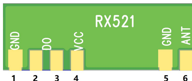
图 1 RX521 管脚示意图
