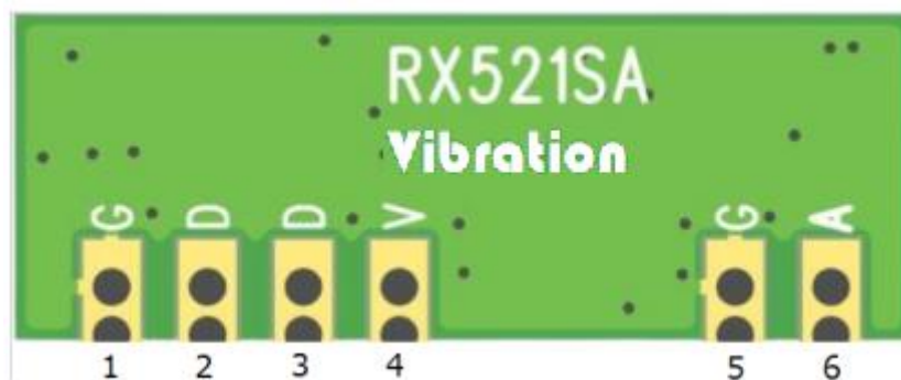
图 1 RX521SA 管脚示意图
