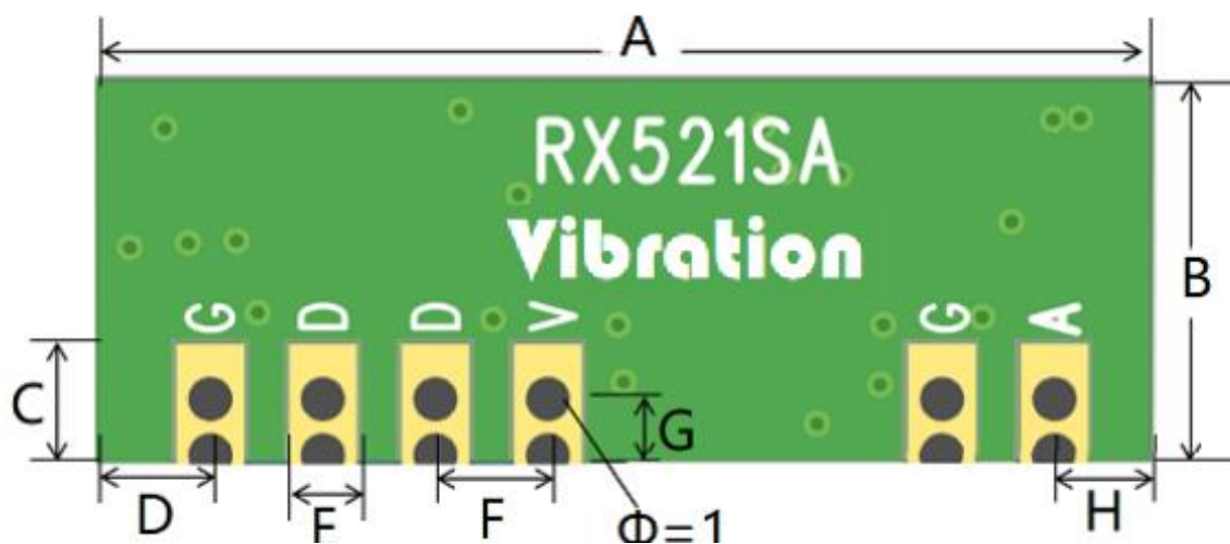
图 2 RX521SA 尺寸示意图
