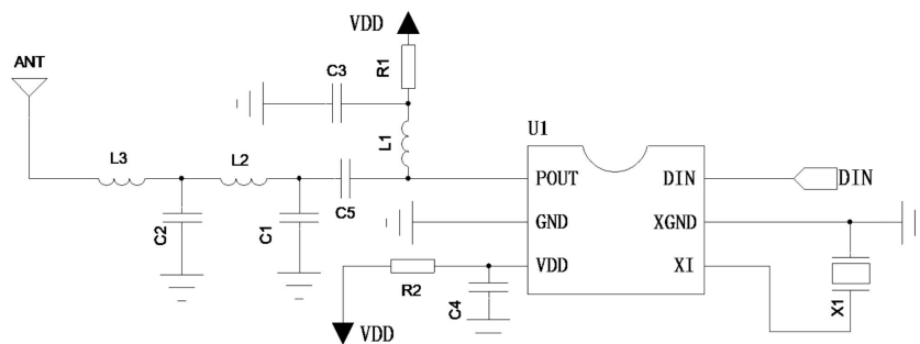
图 3 VI117T 典型应用电路 1
