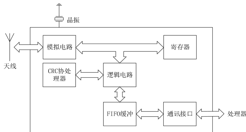
图 2 VRC522B 内部电路框架图
