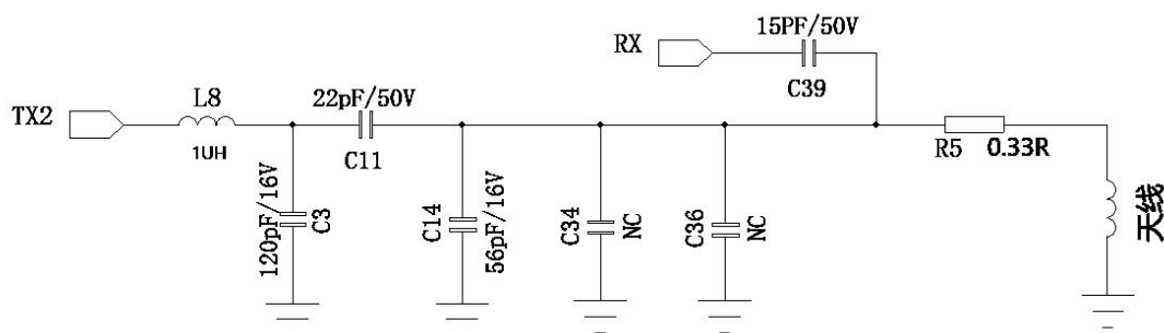
图 7 VRC522B 单线圈天线匹配原理图
