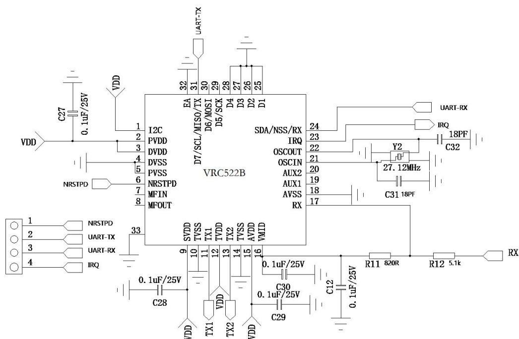
图 5 VRC522B UART 接口应用电路图
