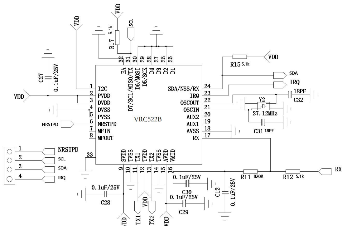
图 4 VRC522B IIC 接口应用电路图
