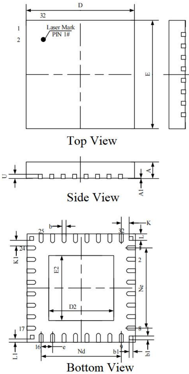
图 8 QFN32 封装示意图
