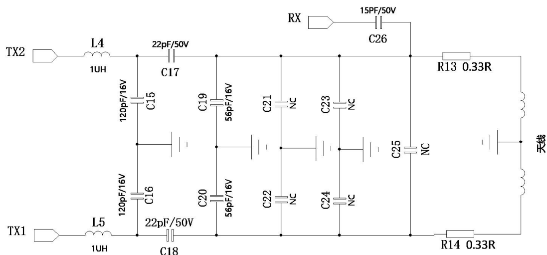
图 6 VRC522B 双线圈天线匹配原理图
