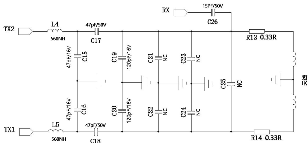
图 6 VRC522 双线圈天线匹配原理图
