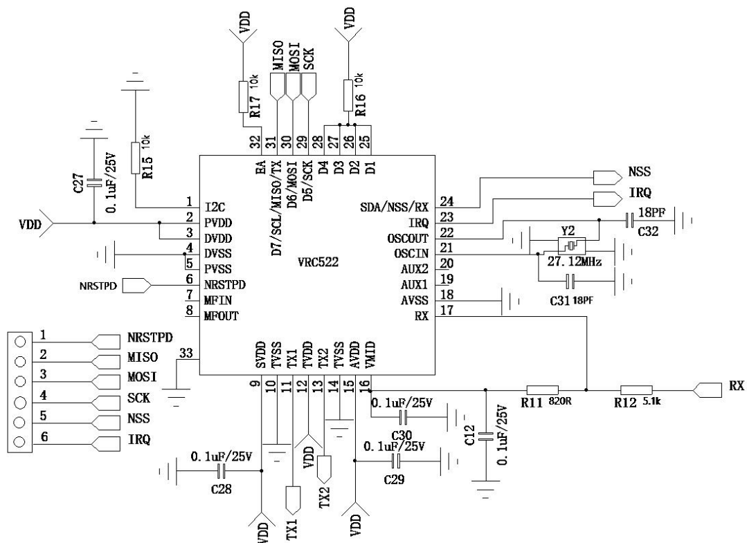
图 3 VRC522 SPI 接口应用电路图
