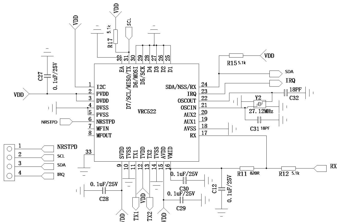
图 4 VRC522 IIC 接口应用电路图
