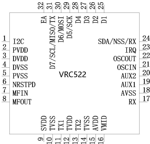
图 1 VRC522 管脚示意图
