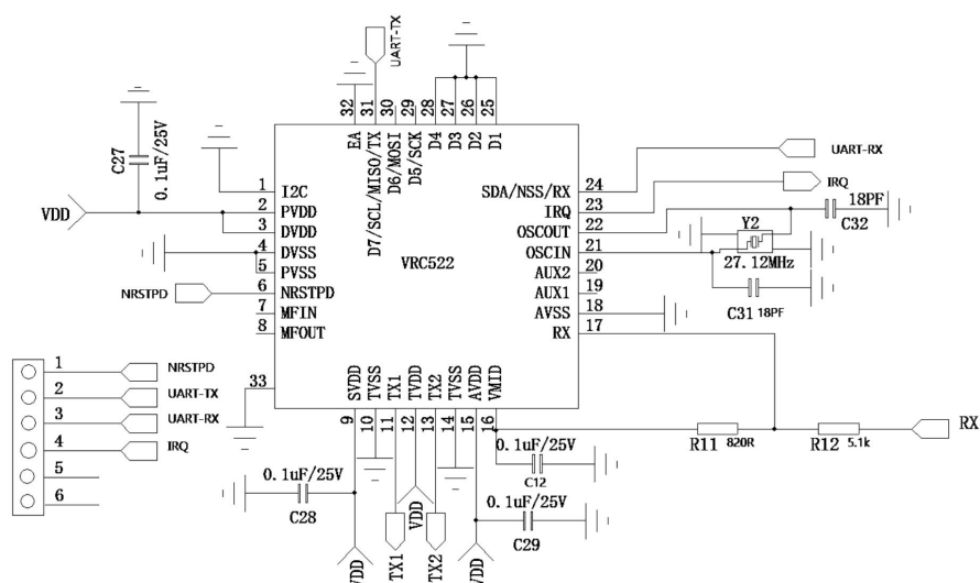
图 5 VRC522 UART 接口应用电路图
