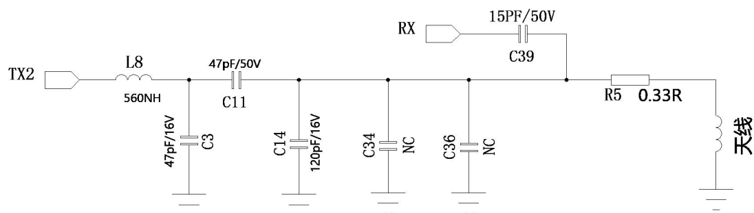
图 7 VRC522 单线圈天线匹配原理图
