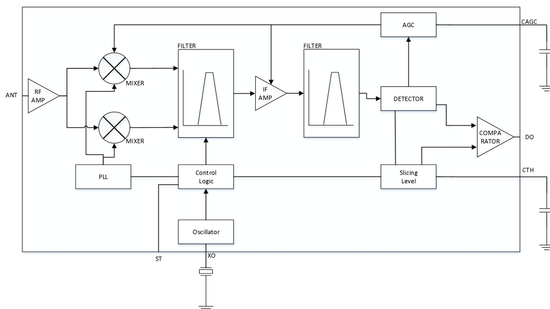
图 2 VT231R 内部电路框架图
