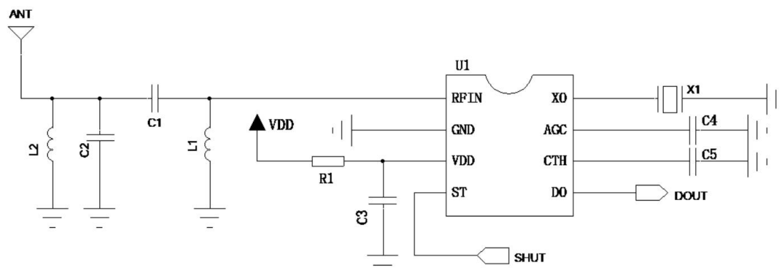
图 3 VT231R 典型应用电路
