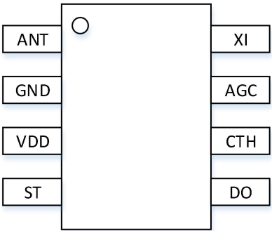
图 1 VT231R 管脚示意图
