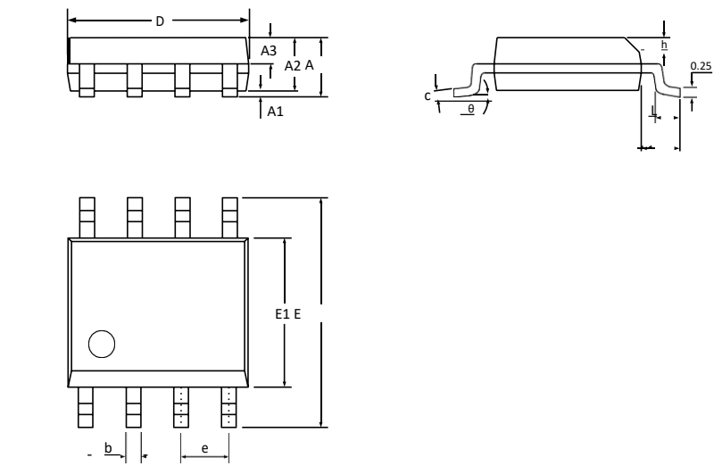
图4. SOP8 封装
