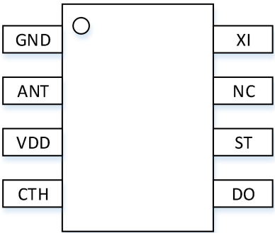
图 1 VI521R 管脚示意图
