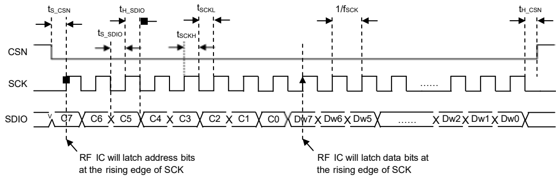
3 线 SPI 接口写入 1 个字节数据
