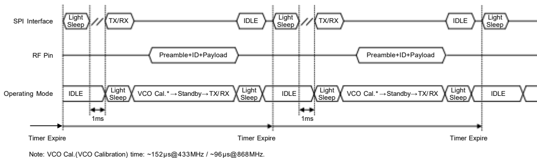
周期性 TX/RX 时序
