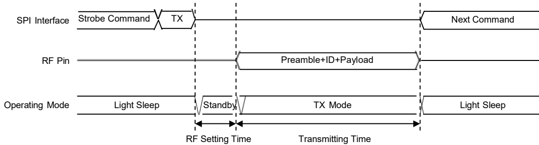
FIFO 模式 TX 时序图
