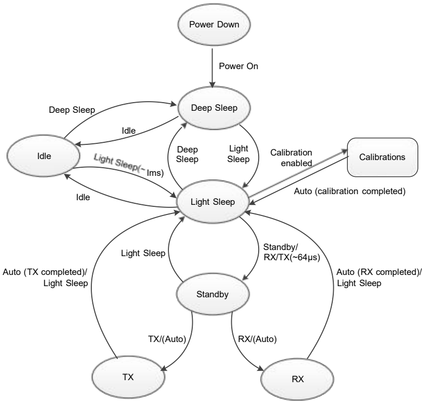
FIFO 模式状态方框图
