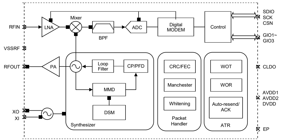
方框图
